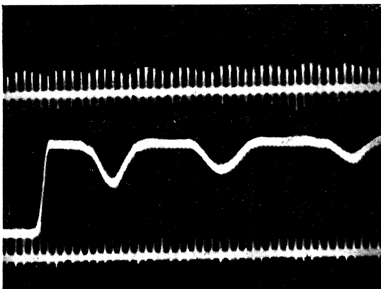
Obr. 2. Oscilogram otevření uzávěrky komory NAFA 3c/25; signál pro kalibraci má frekvenci 500 Hz. Na oscilogramu je vidět vibrační části uzávěrky po otevření.
