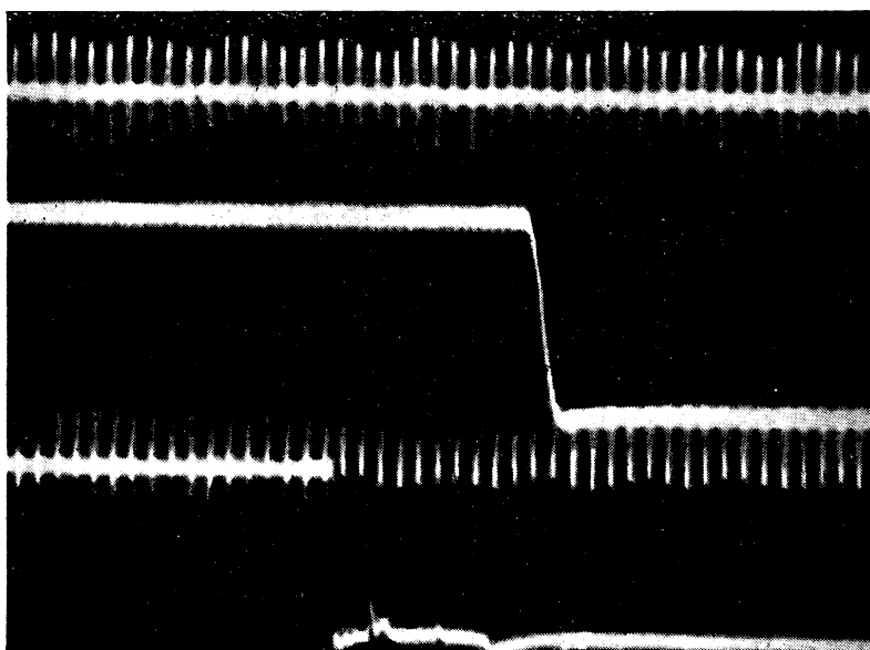
Obr. 3. Oscilogram zavření uzávěrky komory NAFA 3c/25.
