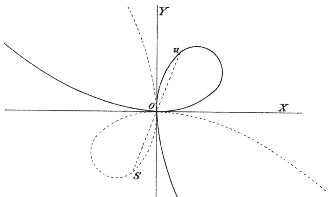
Obrázek 9. Zahradníková konstrukce geometrického místa průsečíků težnic osculačních trojic
