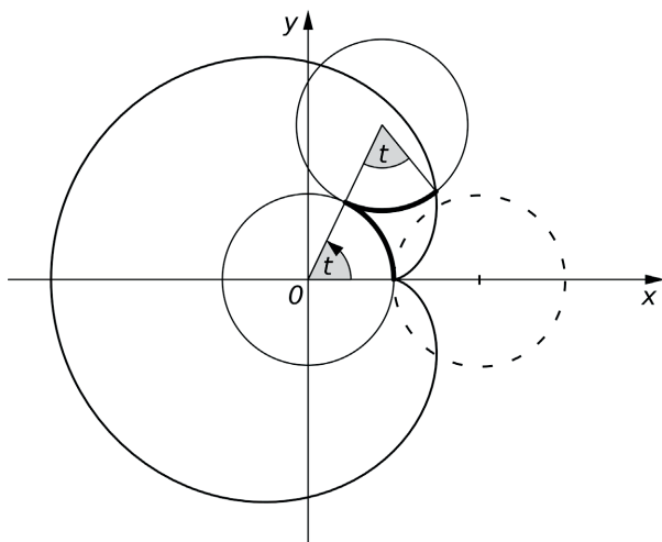
Obrázek 6. Kardioida
