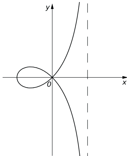
Obrázek 8. Strophoida
