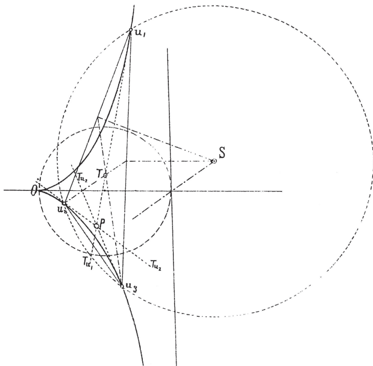
Obrázek 2. Zahradníkova konstrukce
