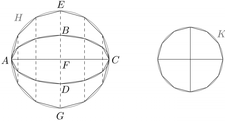
Obr. 4: Archimédův důkaz využívající osovou afinitu
