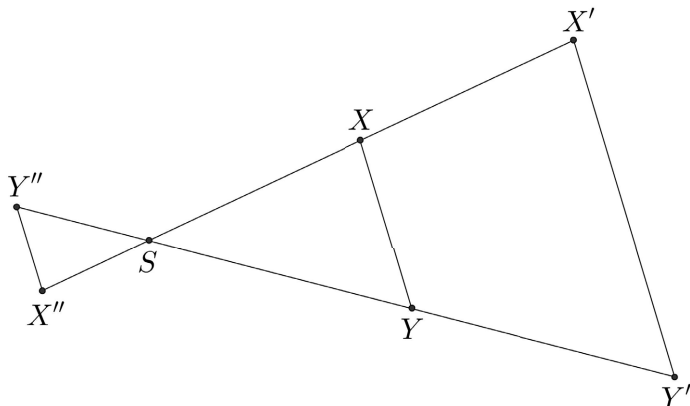
Obr. 5: Stejnolehlosti se středem S a koeficienty \kappa_1 = 2 a \kappa_2 = -\frac{1}{2}
