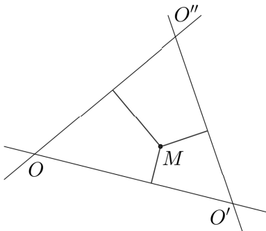
Obr. 26: Trilineární souřadnice
