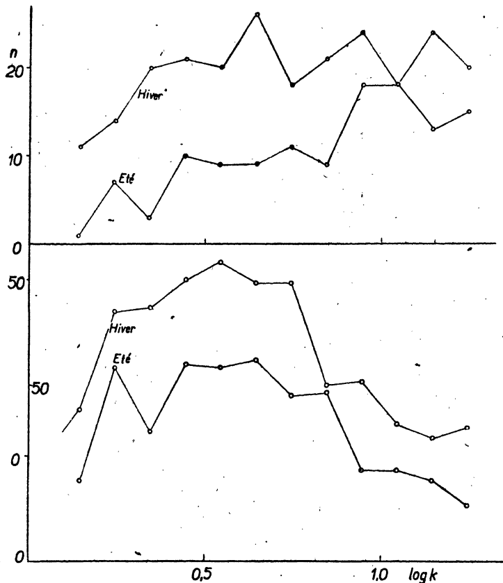
Fig. 3. Statistique des rapports k pour les météores brillants (en haut) et les météores faibles (en bas). L'intervalle de \log k est le double de celui de la fig. 2.
