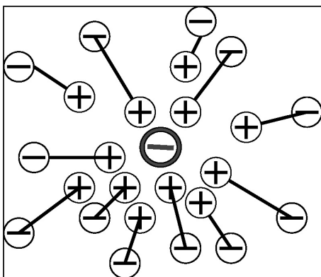
Obr. 5. Polarizace vakua v kvantové elektrodynamice v důsledku vložení záporného holého náboje (tučný kroužek).
