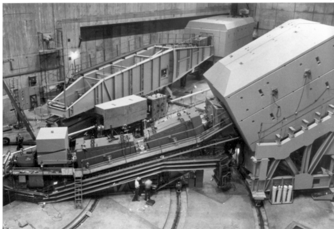
Obr. 13. Schematické uspořádání experimentu, v němž byly ve SLAC rozptýlovány elektrony na protonech (nahore) a ramena spektrometru, která umožňovala měřit úhly a energie rozptýlených elektronů.
