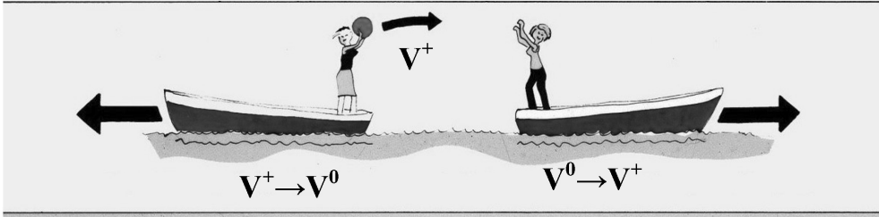
Obr. 9. Síly působící mezi třemi zprostředkujícími vektorovými bosony v teorii Yanga a Millse jsou zprostředkovány výměnou stejných vektorových bosonů jako síly mezi nukleony.
