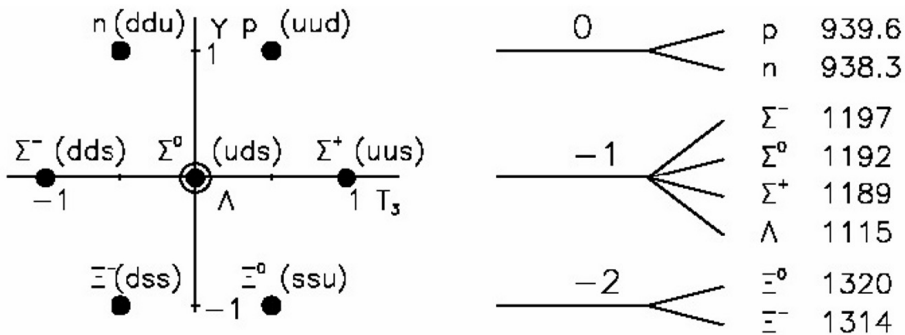
Obr. 10. Oktet baryonů se spinem \frac{1}{2} , do nějž patří také proton a neutron. Částice ležící na vodorovných přímkách mají stejnou hodnotu kvantového čísla, jemuž se říká podivnost, a blízké hmotnosti. Rozdíly hmotností mezi různými „patry“ jsou ovšem podstatně větší. Z hlediska jaderných sil představují všechny částice přitom jen různé stavy jednoho hyperonu. Symboly v závorkách specifikují kvarkové složení, o němž bude řeč dále.
