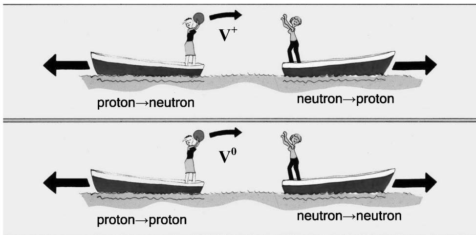
Obr. 8. Mechanická analogie mechanismu jaderných sil v systému tvořeném protonem a neutronem v teorii Yanga a Millse. Na horním obrázku proces „nábojové výměny“, při němž se proton mění na neutron a obráceně, dole pružný rozptyl, zprostředkovaný výměnou neutrálního vektorového bosonu V^0 .
