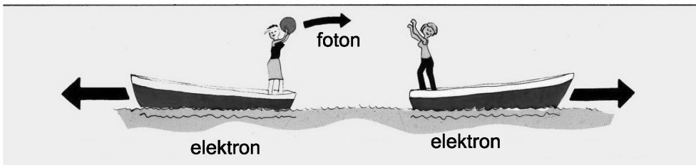
Obr. 7. Mechanická analogie mechanismu elektromagnetických sil působících mezi dvěma elektrony v kvantové elektrodynamice. Protože foton má nulovou klidovou hmotnost, „dohodíme“ s ním do nekonečna a elektromagnetické síly mají proto daleký dosah. Tímto způsobem lze ovšem jednoduše modelovat jen odpudivé síly.
