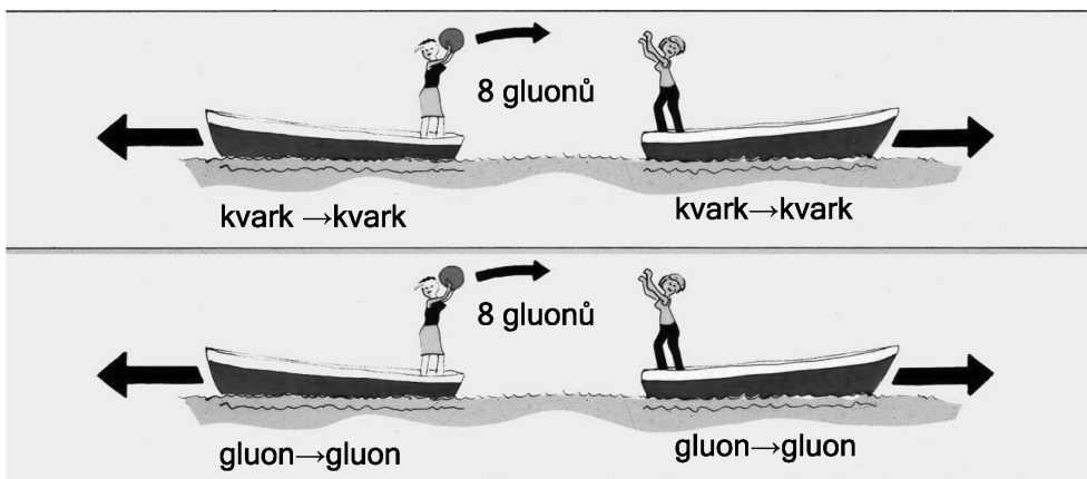
Obr. 12. Grafické znázornění mechanismu sil působících mezi dvěma kvarky (nahore) a dvěma gluony (dole) zprostředkované výměnami osmi barevných gluonů. Při výměnách se obecně mění barva kvarků a gluonů-loděk, ale tak, že při každém aktu „odhození“ gluonu se barva zachovává.
