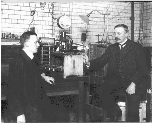
Obr. 3. Vlevo: Rutherford s Marsdenem u svého zařízení, jehož schéma je znázorněno vpravo. Částice alfa vycházející ze zdroje R se rozptýlily na zlaté fólii F a dopadaly na vrstvu ZnS na předním okénku kukátka M, které se otáčelo kolem osy kolmé na rovinu obrázku a do nějž se dívali střídavě Geiger s Marsdenem.
