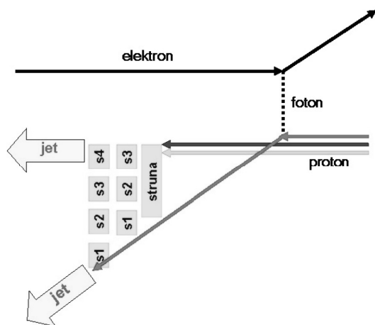
Obr. 14. Feynmanova představa o průběhu tvrdé srážky elektronu s protonem, jehož výsledkem jsou dva jety.
