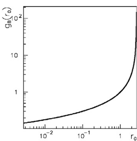
Obr. 15. Závislost holého barevného náboje g_B na jeho poloměru r_0 , zajišťující konečnost efektivního barevného náboje g(r) .
