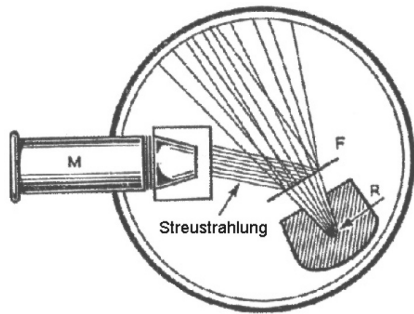
Obr. 3. Vlevo: Rutherford s Marsdenem u svého zařízení, jehož schéma je znázorněno vpravo. Částice alfa vycházející ze zdroje R se rozptýlily na zlaté fólii F a dopadaly na vrstvu ZnS na předním okénku kukátka M, které se otáčelo kolem osy kolmé na rovinu obrázku a do nějž se dívali střídavě Geiger s Marsdenem.
