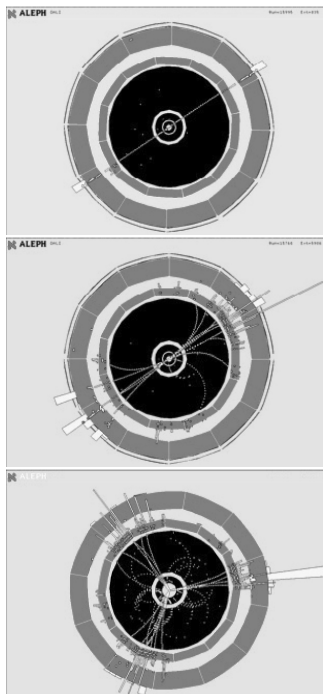
Obr. 17. Srovnání produkce mionů a jetů ve srážkách elektronů s pozitrony.
